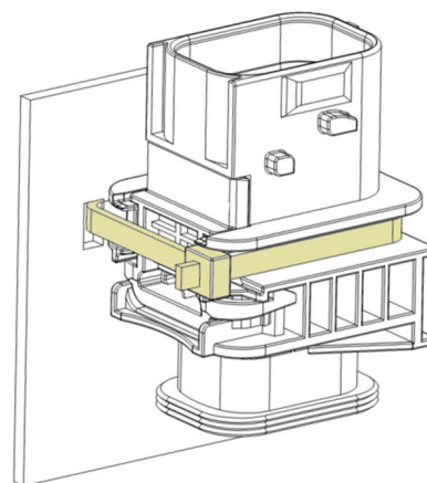
Рисунок 7. Крепление разъема.
