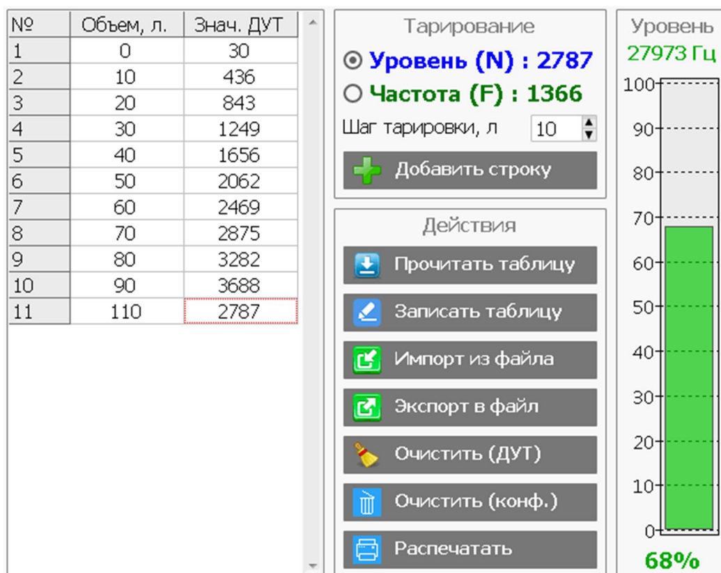
Рисунок 14. Тарирование.
