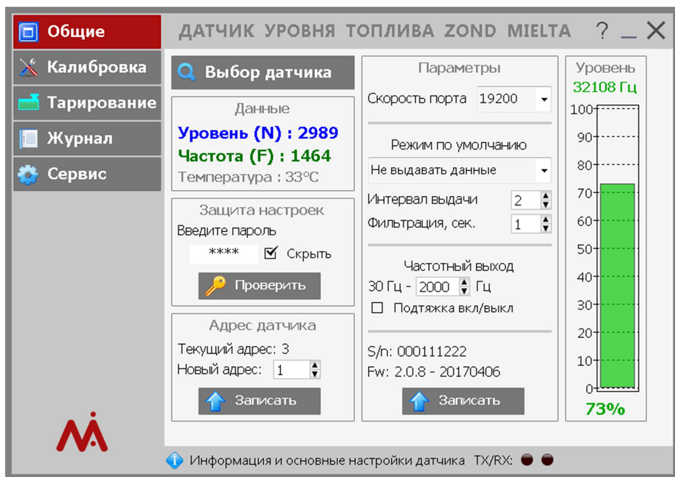
Рисунок 11. Главное окно программы-конфигуратора
