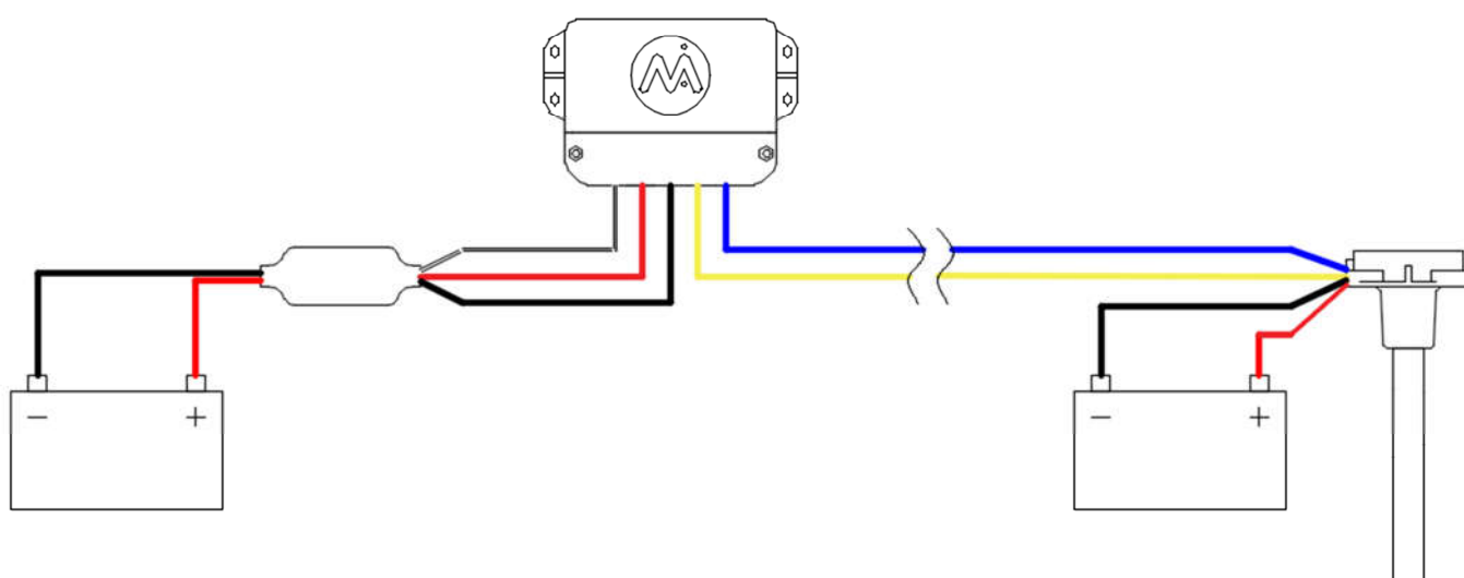
Рисунок 10. Схема подключения по интерфейсу RS485 и отдельными источниками питания.
