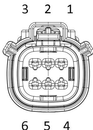
Рисунок 6. Нумерация контактов в разъеме ДУТ.
