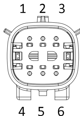
Рисунок 7. Нумерация контактов в разъеме жгута.
